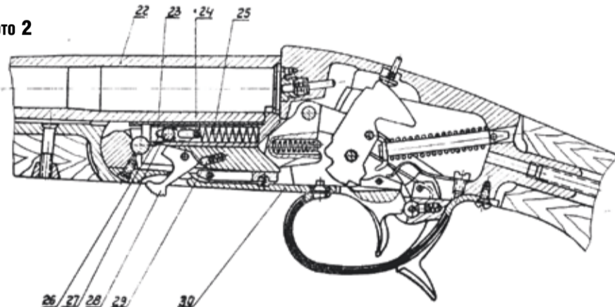
Рис. 2. Схема механизмов ружья ИЖ-18Е. 22 — Ствол. 23 — Экстрактор. 24 — Штифт опорный. 25 — Пружина экстрактора. 26 — Фиксатор штифта. 27 — Штифт экстрактора. 28 — Шептало экстрактора. 29 — Гнеток. 30 — Личинка.
