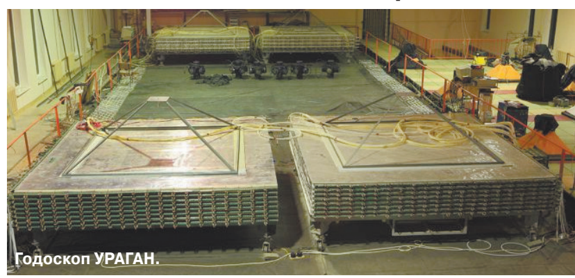
Годоскоп УРАГАН.
