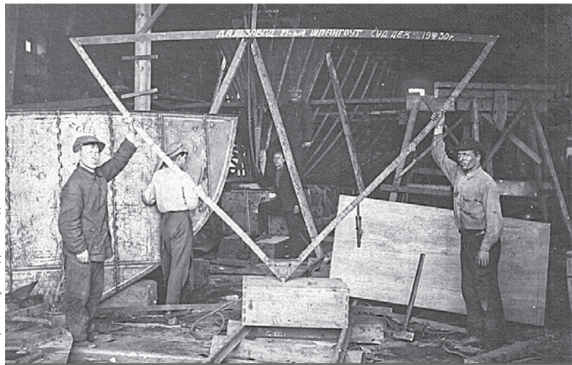
Набор шпангоута первого цельносварного катера.
